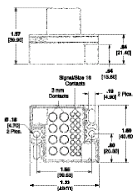
Receptacle 194299-1
