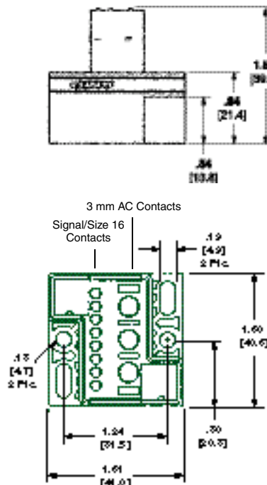
Receptacle 194279-1
