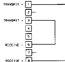
Wiring Schematic
