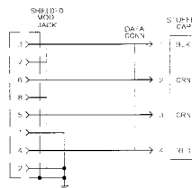
Token Ring Wiring
