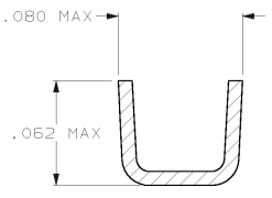
SECTION A-A SCALE 20:1
