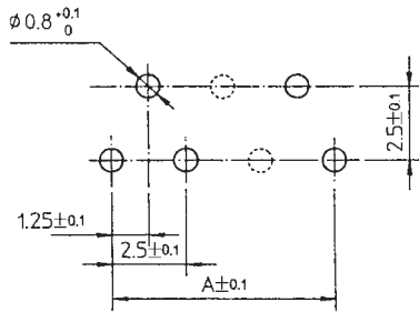
基板穴寸法 (コネクタ略観面) MOUNTING LAYOUT (適用基板厚 t=1~1.6) (t=1~1.6)
