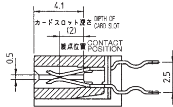
奇数ピン位置 EVEN PIN POSITION
