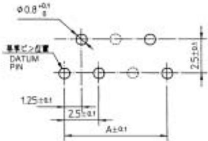
標準穴径寸法 (コネクタ標準値) MOUNTING LAYOUT (適用厚板厚 1~1.6) (t=1~1.6)
