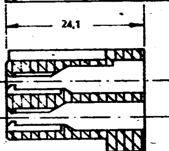
SCHNITT A-A
