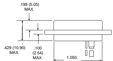
Receptacle
