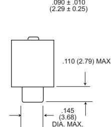
Receptacle
