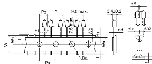
BL02RN2R1□1A
