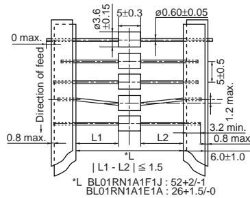
BL01RN_A
