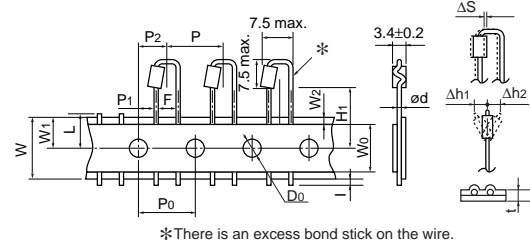
BL02RN2R1□1A
