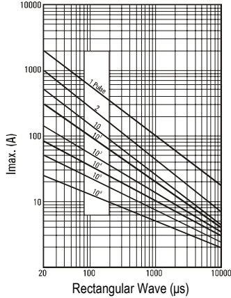
ROV14H820K – ROV14H511K
