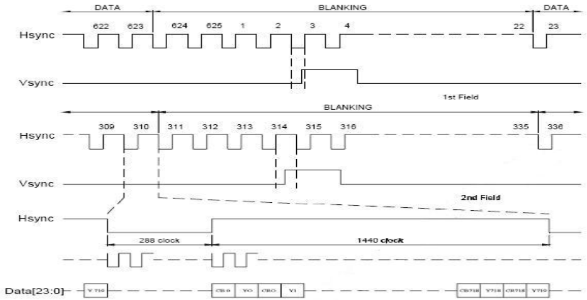
ITU-BT 601 PAL Input Timing
