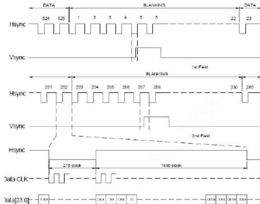
ITU-BT.601 NTSC Input Timing
