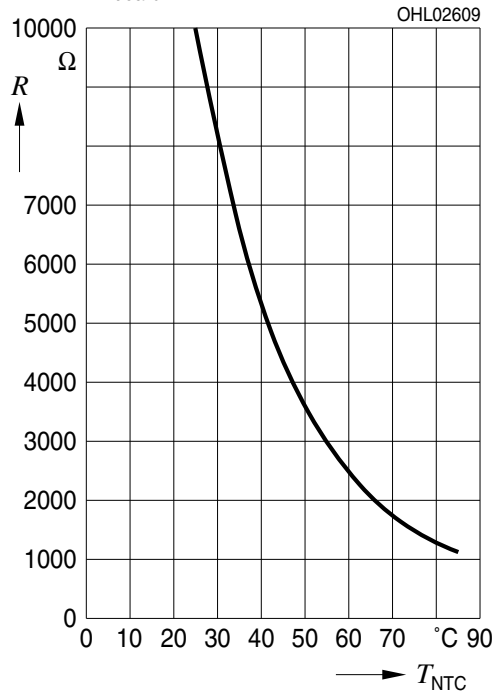
Typische Thermistor Kennlinie 2) 5) Seite 19 Typical Thermistor Graph 2) 5) page 19
