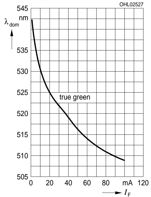
Dominante Wellenlänge 6) Seite 22 Dominant Wavelength 6) page 22 true green, \lambda_{\text{dom}} = f(I_F); T_A = 25 \text{ }^\circ\text{C}
