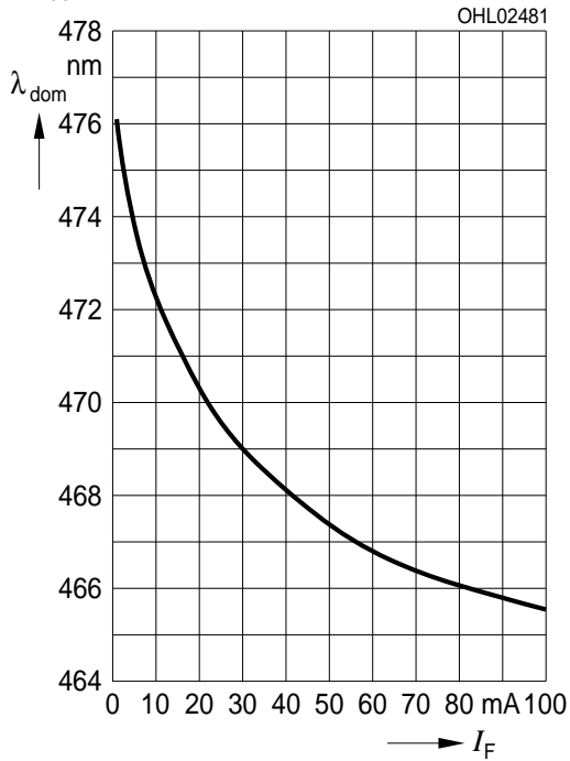
Dominante Wellenlänge 6) Seite 22 Dominant Wavelength 6) page 22 blue, \lambda_{\text{dom}} = f(I_F); T_A = 25 \text{ }^\circ\text{C}
