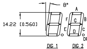
DIGIT DETAIL
