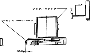
断面 C-C (尺度: 2-1)
