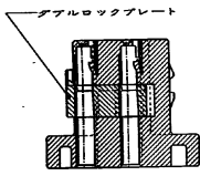
断面 A-A (尺度: 2-1)
