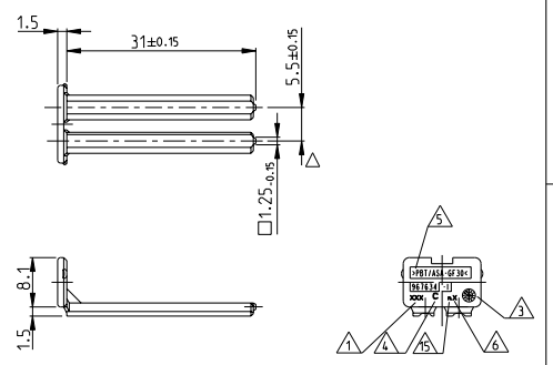
967634-1 AS SHOWN wie gezeichnet
