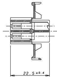
SECTION A-B
