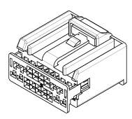
638116-2 KEY B CONFIGURATION SCALE: 2:1
