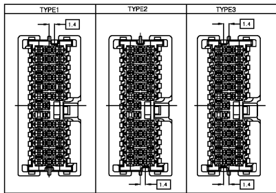
SECTION A-A <KEY CODE>
