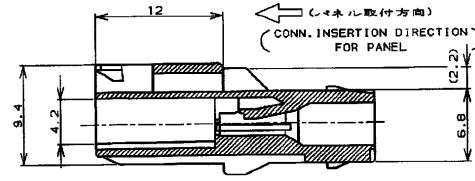
断面 "A-A" (SECT)
