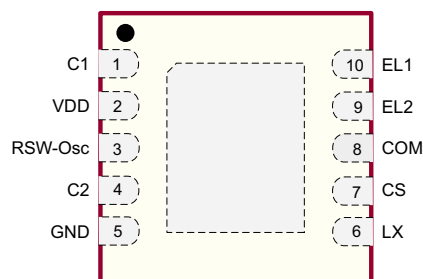
10-Lead DFN (K6)
