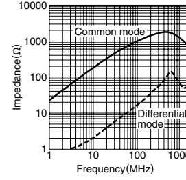
ACM3225-102-2P
