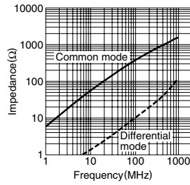
ACM2520-102-2P
