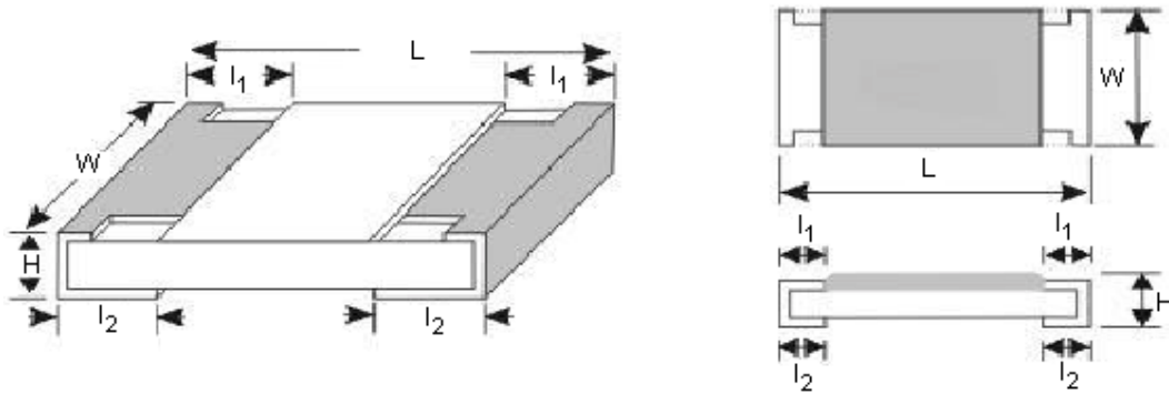
Dimensions : Millimetres
