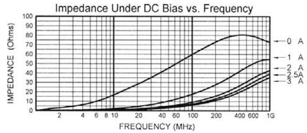
MLB-201209-0060PQ
