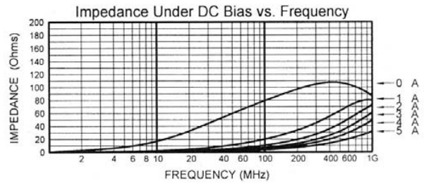
MLB-201209-0080PU
