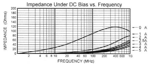
MLB-201209-0090PU
