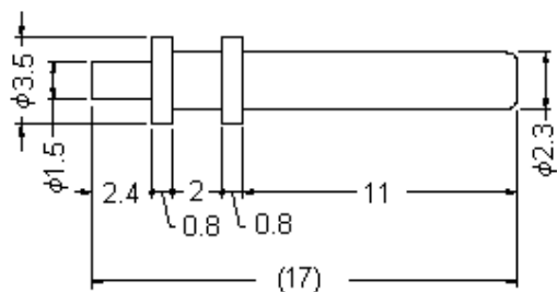
Dimensions : Millimetres
