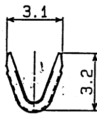
A-A SEC.
