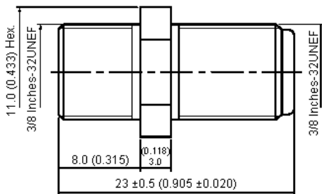
Dimensions : Millimetres (Inches)
