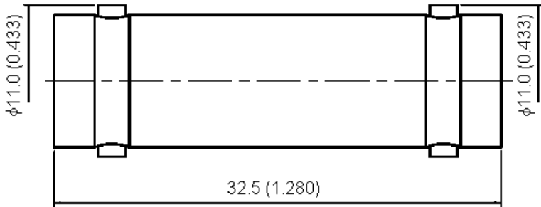
Dimensions : Millimetres (Inches)
