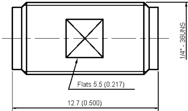
Dimensions : Millimetres (Inches)
