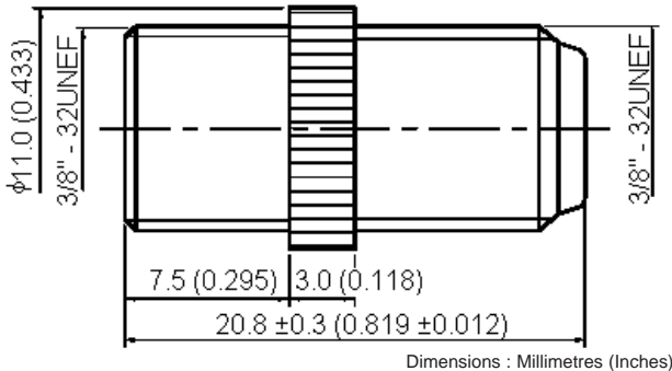
Dimensions : Millimetres (Inches)
