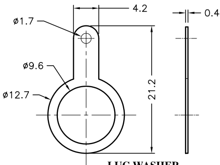
LUG WASHER
