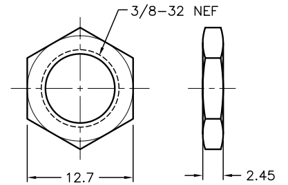
NUT
