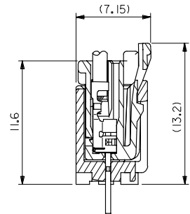
嵌合断面図
