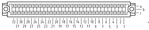
X Kontaktbelegung contact loading
