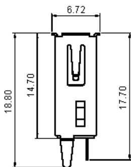
Dimensions : Millimetres
