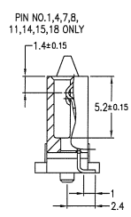
SECT-X-X
