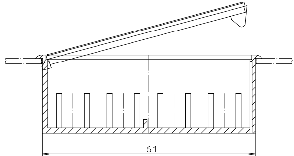
Einbauöffnung BE 60
