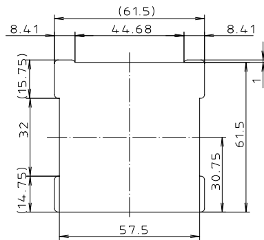
Einbauöffnung BE 60
