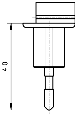
Euro-Stecker 1717707 Euro-plug 1717707
