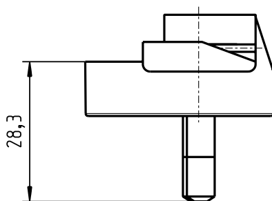
Australien-Stecker 1800496 Australian-plug 1800496
