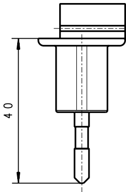
Euro-Stecker 1717707 Euro-plug 1717707
