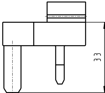
UK-Stecker 1717618 UK-plug 1717618
