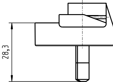
Australien-Stecker 1800496 Australian-plug 1800496
