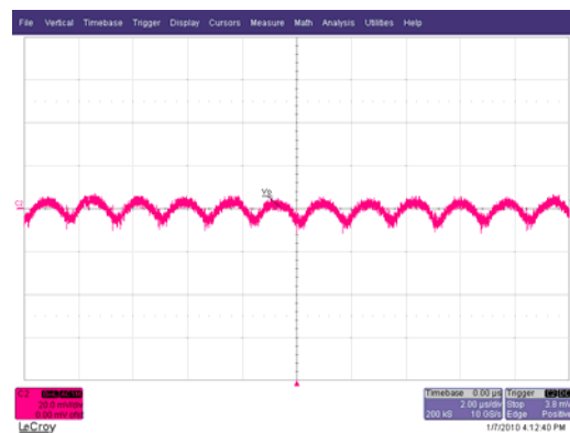
Fig. 10. Output Voltage Ripple, 3A load Ch 2 : V o
