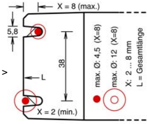
Befestigungs-Maße
