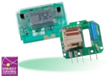
MEU11/EMU17 PB05
