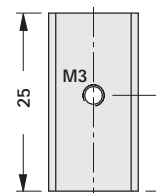
SK 95 25 SOT 32
