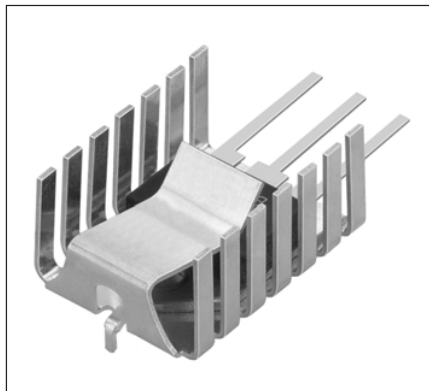
FK 243 MI 247 H 19 K/W mit Lötflanke für horizontalen Einbau with solder lug for horizontal installation
