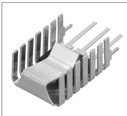
FK 243 MI 247 V 18,4 K/W mit Lötflanke für vertikalen Einbau with solder lug for vertical installation
