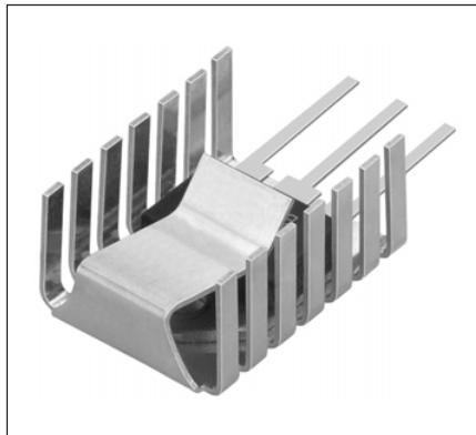
FK 243 MI 247 O 18,7 K/W ohne Lötflanke without solder lug
