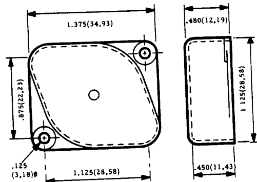
ME 415/TO 3 FLANGE
