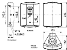
Bauzeichnung
