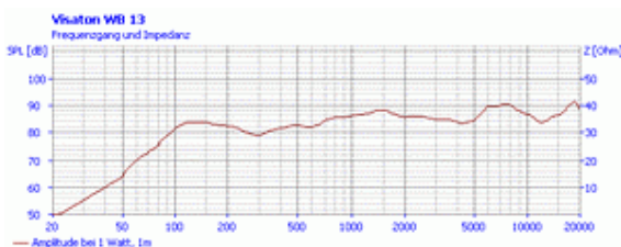
Amplitudenfrequenzgang
