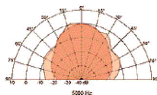
Abstrahlcharakteristik 5000 Hz
