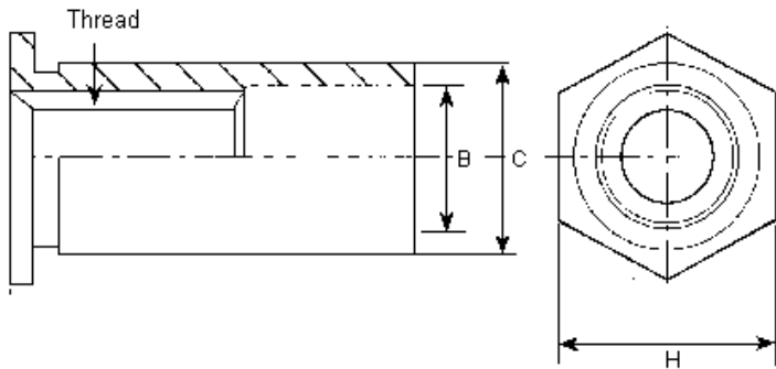
Dimensions : Millimetres
