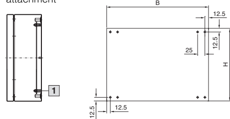
1 Spacer bolts M5 x 15
