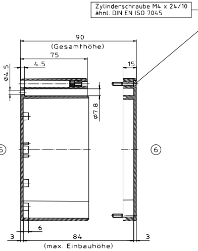
(max. Einbauhöhe)
