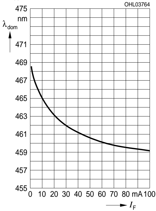
Dominante Wellenlänge 6) Seite 25 Dominant Wavelength 6) page 25 blue, \lambda_{\text{dom}} = f(I_F); T_A = 25\text{ °C}
