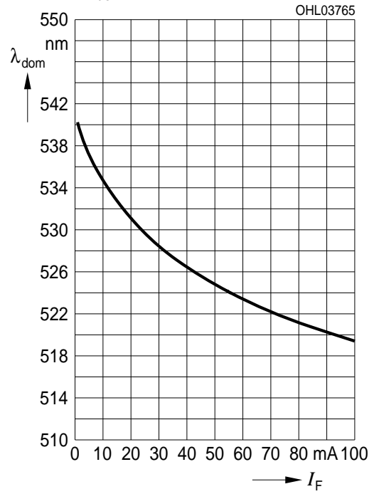
Dominante Wellenlänge 6) Seite 25 Dominant Wavelength 6) page 25 true green, \lambda_{\text{dom}} = f(I_F); T_A = 25\text{ °C}
